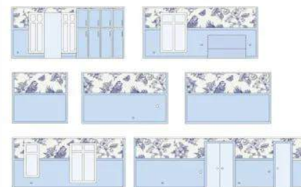
Разработка стен в спальне 2 этажа
