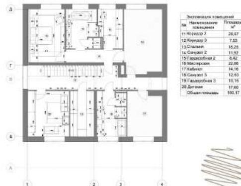
План мебели (вариант 3. Итоговый) 2 этаж
