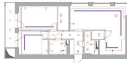
ПЛАН РАСТАНОВКИ ОБЪЕКТНОГО ОБОРУДОВАНИЯ №150
