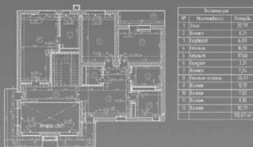
План перепланировки 2-го этажа М 1:100
